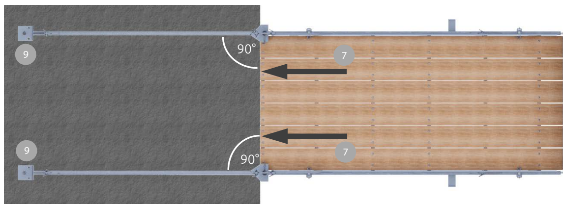
Variante de fixation 1 avec 1 étai de dalle + fixation par longeron porteur
