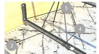
System Randfix mit Elementdecken und Randfix Halter.
