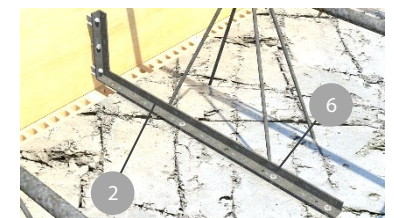
System Randfix mit Elementdecken und Nageldübel.
