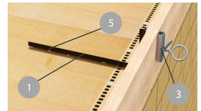
System Randfix bei Deckenschalung aus Holz.
